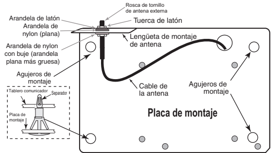
Figura 1: Soporte de montaje del Comunicador
