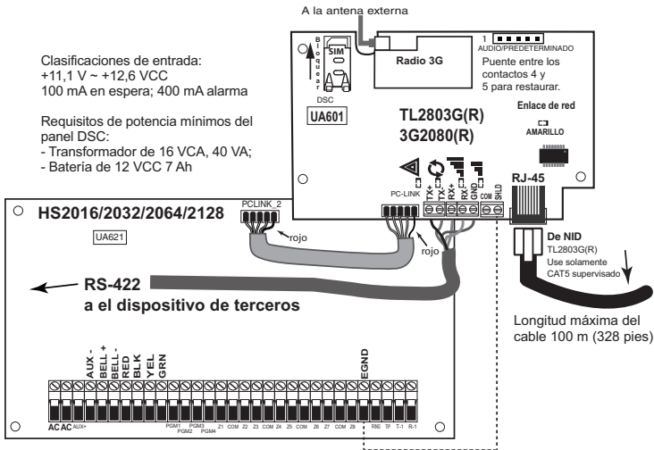
Figura 3: Diagrama de cableado del Comunicador
